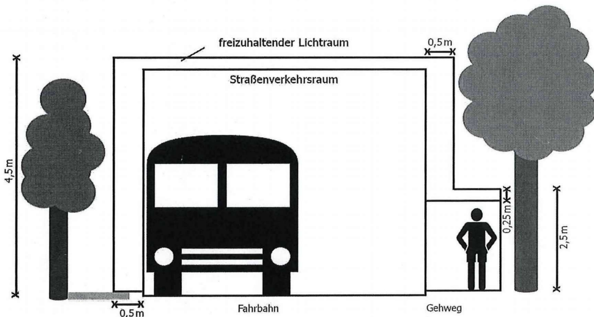
Grafik: Straßenlichtraumprofil, das von Bewuchs freizuhalten ist
